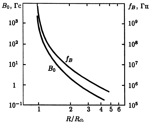
Рис. 2. Распределение магнитного поля B_0 и гирочастоты f_B на оси униполярного солнечного пятна с B_b = 2.5 \cdot 10^3 Гс и b = 10^{19} см
