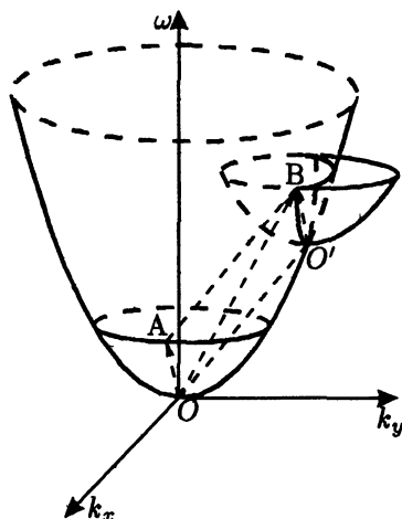
Рис. 68. Критерий распадного спектра
