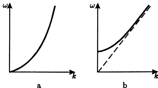
Рис. 67. Примеры распадного (а) и нераспадного (б) спектров
