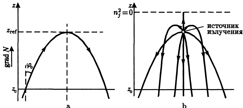
Рис. 19. Рефракция в плоскослойной плазме с \nabla N вдоль оси z : (а) форма луча, входящего в плазму под углом \varphi_0 ; (б) лучи от точечного источника в плазме
