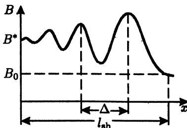
Рис. 47. Профиль ударной волны в плазме
