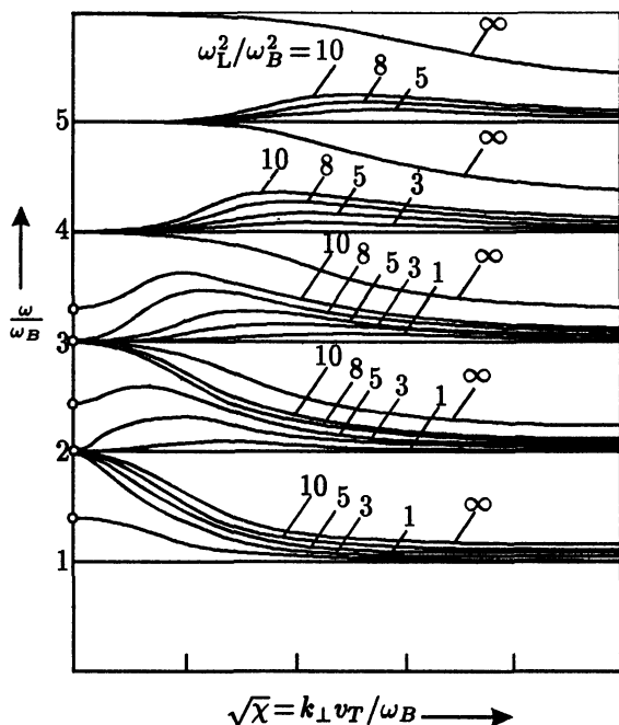
Рис. 14. Дисперсионные кривые для мод Бернштейна в нерелятивистской равновесной плазме. Светлыми точками на оси \omega/\omega_B отмечены значения, где \omega = \omega_h
