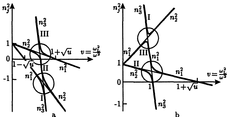
Рис. 13. Дисперсионные кривые n_j^2(v) ( j = I, II, III ) при учете теплового движения в плазме ( \alpha \ll 1 ): (а) u < 1 ; (б) u \cos^2 \alpha > 1 . Кружками указаны области взаимодействия волн в неоднородной плазме, тонкими линиями внутри кружков — зависимость n_j^2(v) в случае продольного распространения
