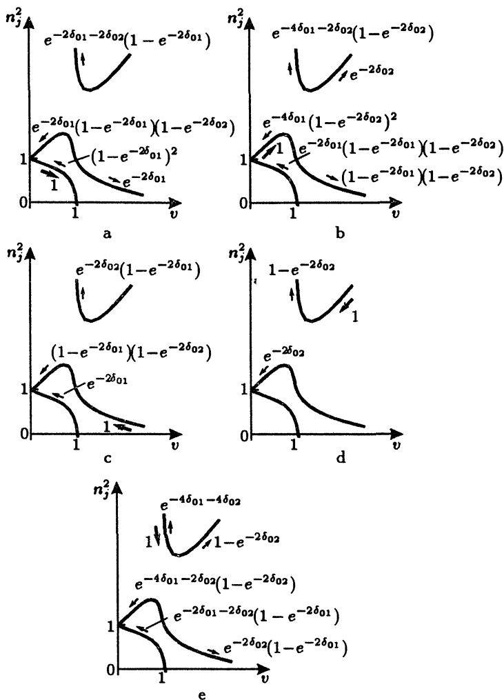
Рис. 33. Различные варианты линейного взаимодействия при \mu \cos^2 \alpha > 1 . Обозначения те же, что на предыдущем рисунке
