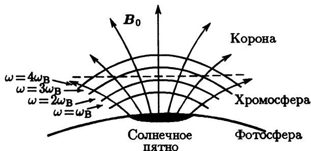
Рис. 44. Расположение гирорезонансных уровней в униполярном магнитном поле
