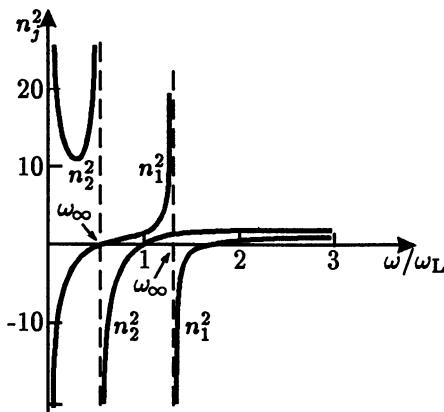
Рис. 11. Дисперсионные кривые n_j^2(\omega) при постоянных \omega_L и \omega_B (для \omega_B/\omega_L=1 и \alpha=\pi/4 )
