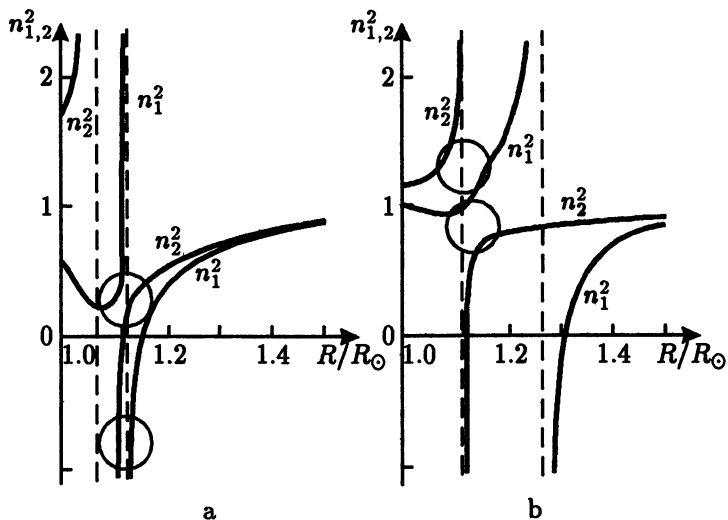
Рис. 17. То же, что и на Рис. 16, для \alpha = 15^\circ . Кружками отмечены области взаимодействия разных типов волн
