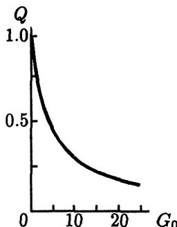
Рис. 30. Коэффициент трансформации Q при прохождении волн через область с нулевым магнитным полем (зависимость от параметра взаимодействия G_0 ), когда волна переходит с дисперсионной кривой II на кривую I
