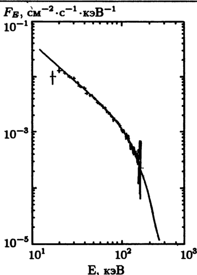
Рис. 59. Сравнение наблюдаемого спектра излучения Cyg X-1 (зависимости спектрального потока фотонов F_E от их энергии E ) со спектром, сформированным в результате комптонизации низкочастотных фотонов в плазменном облаке с \tau_0 = 5 и \kappa T = 27 кэВ [430]
