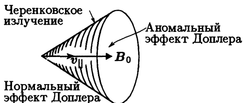
Рис. 37. Области аномального и нормального эффектов Доплера при магнитотормозном излучении электрона в среде. Коническая поверхность соответствует черенковскому излучению
