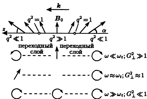
Рис. 22. Распространение волн через область квазиперпендикулярного магнитного поля и изменение их поляризации
