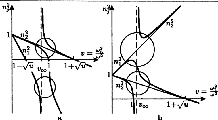
Рис. 10. Зависимость n_j^2(v) при \alpha \ll 1 : (а) u < 1 ; (б) u \cos^2 \alpha > 1 . Кружками отмечены области линейного взаимодействия волн (см. §7)
