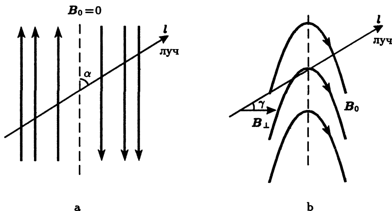
Рис. 28. Конфигурация силовых линий магнитного поля B_0 в случае: (а) нейтрального токового слоя, содержащего поверхность B_0=0 ; (б) токового слоя, представляющего собой суперпозицию полей в нейтральном токовом слое и ортогонального к ним постоянного магнитного поля B_{\perp}
