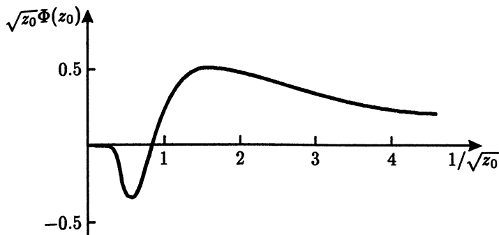
Рис. 57. График зависимости \sqrt{z_0}\Phi(z_0) от 1/\sqrt{z_0}
