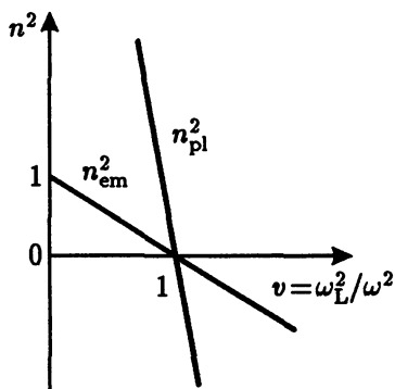
Рис. 7. Зависимость квадрата показателя преломления n_{em}^2 и n_{pl}^2 от параметра v в изотропной плазме
