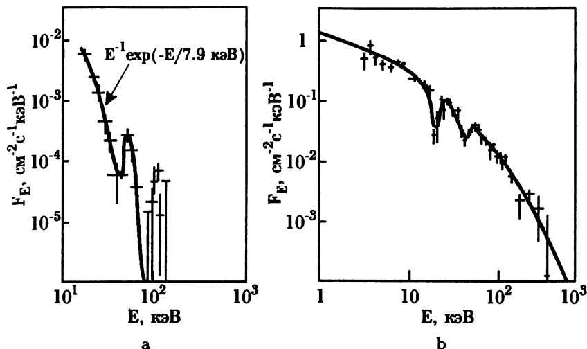
Рис. 63. Спектры рентгеновского излучения (спектральный поток фотонов F_E как функция энергии фотона E ) рентгеновского пульсара Her X-1 (а) [44] и космического гамма-всплеска GB 870303 (б) [446]
