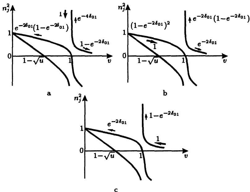
Рис. 32. Различные варианты (а, b и c) линейного взаимодействия волн при u = \omega_B^2 / \omega^2 < 1 . Указаны квадраты модулей амплитуд волн, выходящих из области взаимодействия, при падении на нее волны с единичной амплитудой. Жирной стрелкой отмечена падающая волна, тонкими стрелками — волны, возникающие в результате взаимодействия
