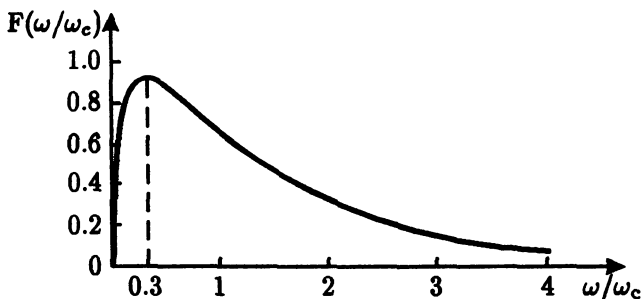
Рис. 39. Частотный спектр синхротронного излучения электрона в вакууме
