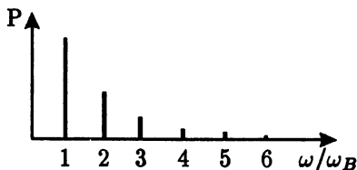
Рис. 38. Частотный спектр циклотронного излучения электрона в пустоте
