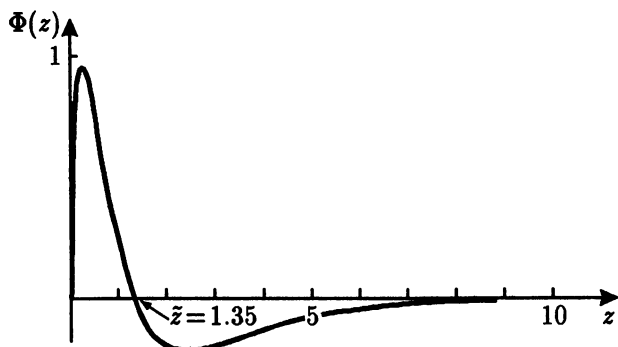
Рис. 56. График функции \Phi(z)
