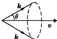
Рис. 36. Конус волновых векторов при эффекте Вавилова – Черенкова
